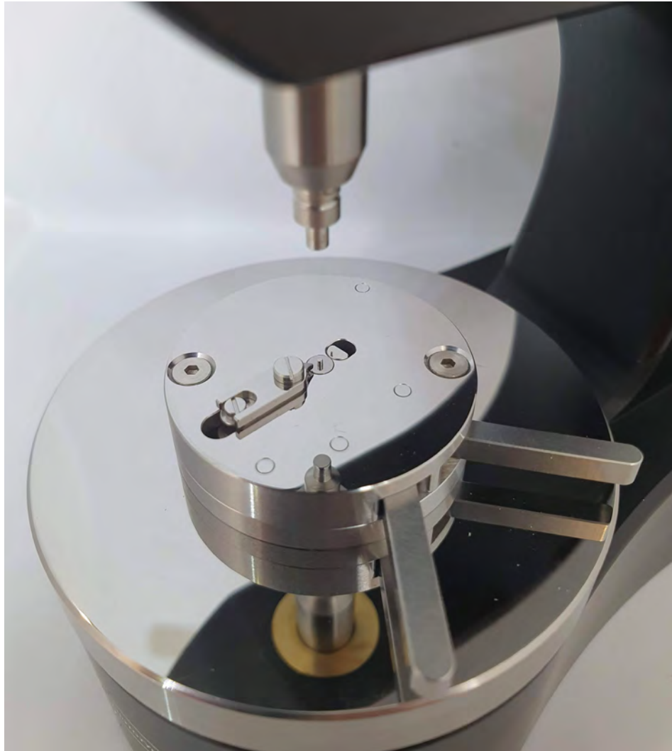
Entwickelt und produziert von Chatelain Prototypes: Montagewerkzeug für das Satellitenrad eines Uhrwerks.
